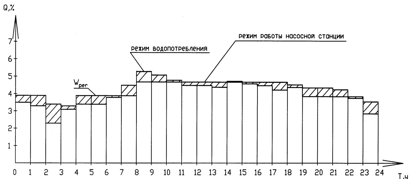
Схема 3 График режимов водопотребления и работы насосной станции II-го подъема.
