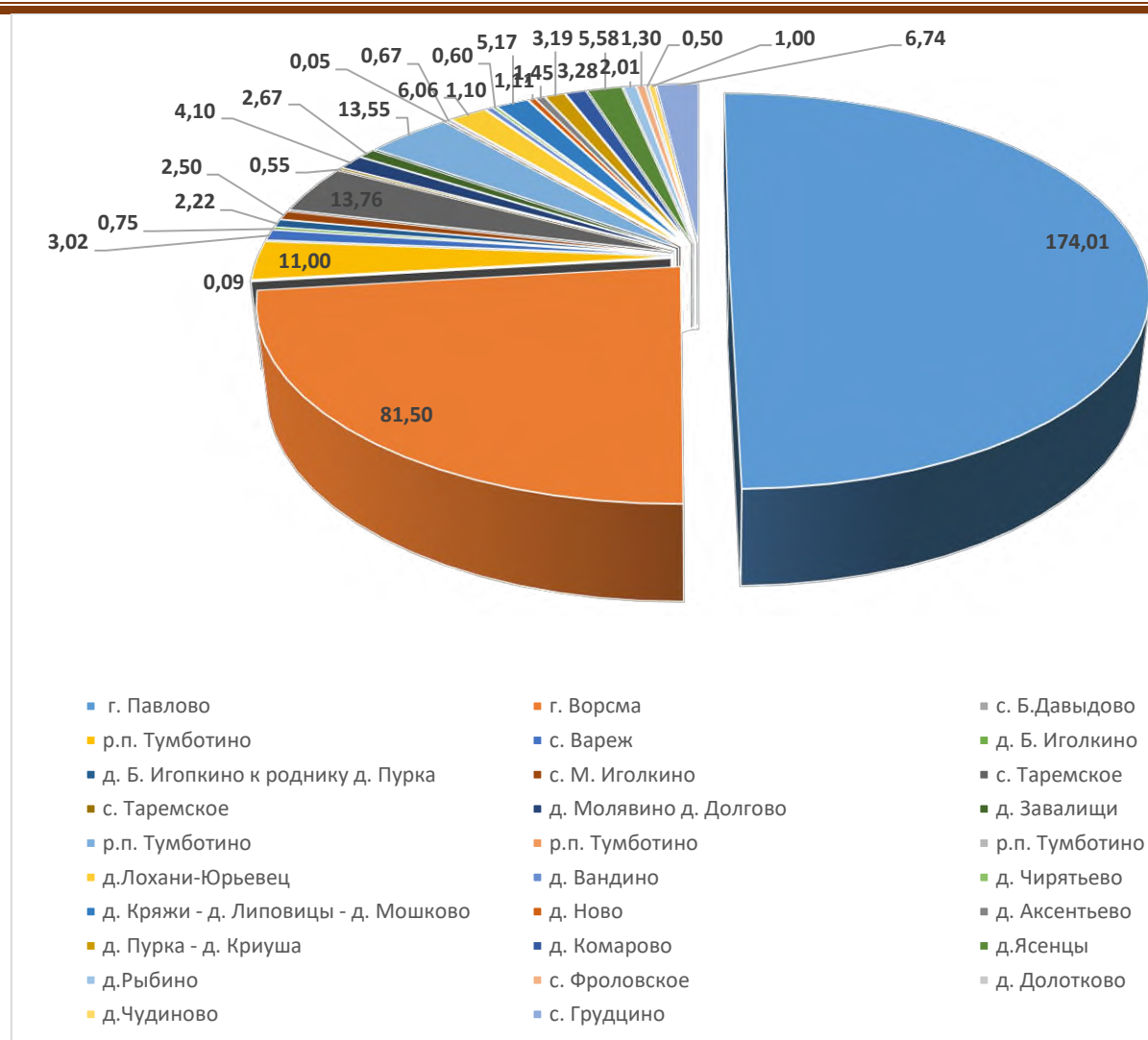
Диаграмма 10 Протяженность водопроводных сетей в зоне деятельности МУП Водоканал г.Павлово, км.
