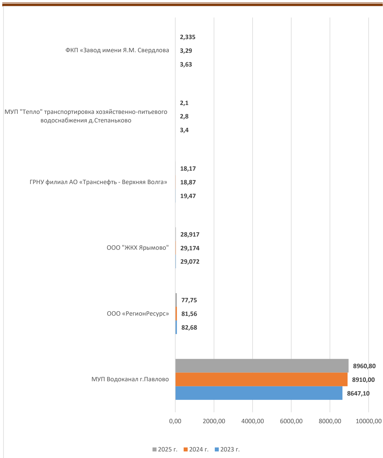
Диаграмма 17 Фактические показатели водоснабжения по РСО за 2023-2025 гг., тыс.м³
