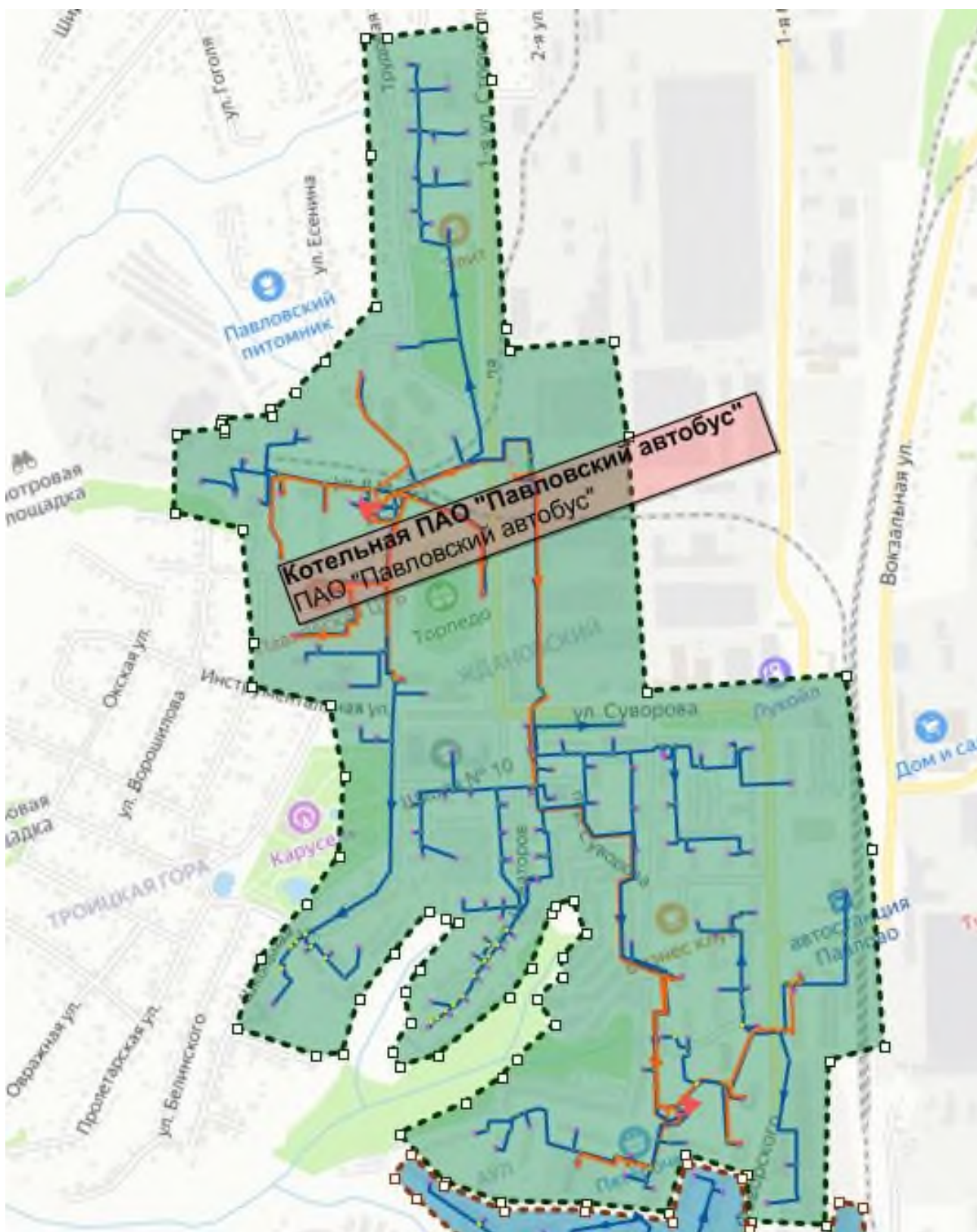
Рисунок 1.7 – Зона действия котельных Павловского муниципального округа.
