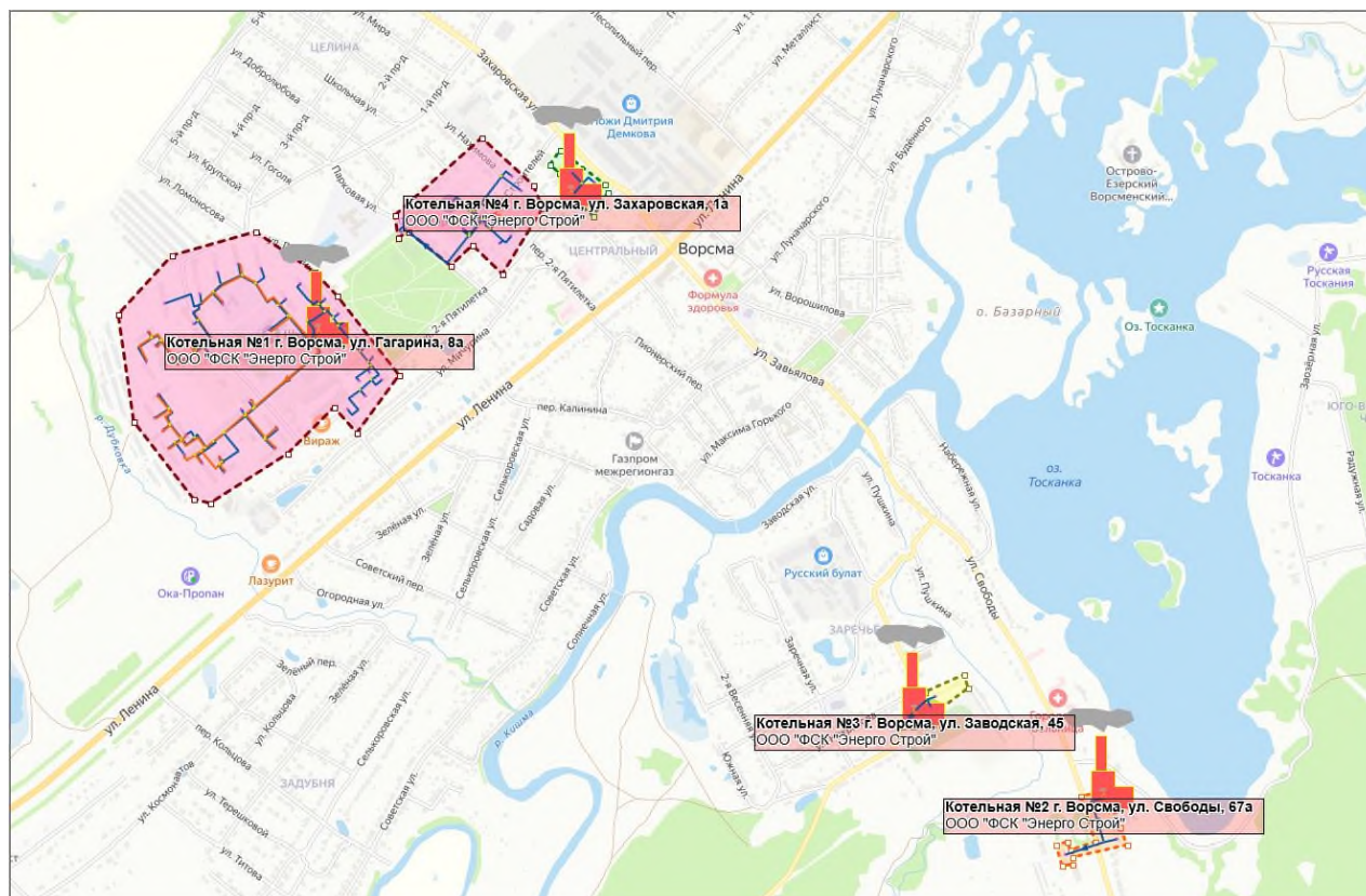
Рисунок 1.10 – Зона действия котельных Павловского муниципального округа.
