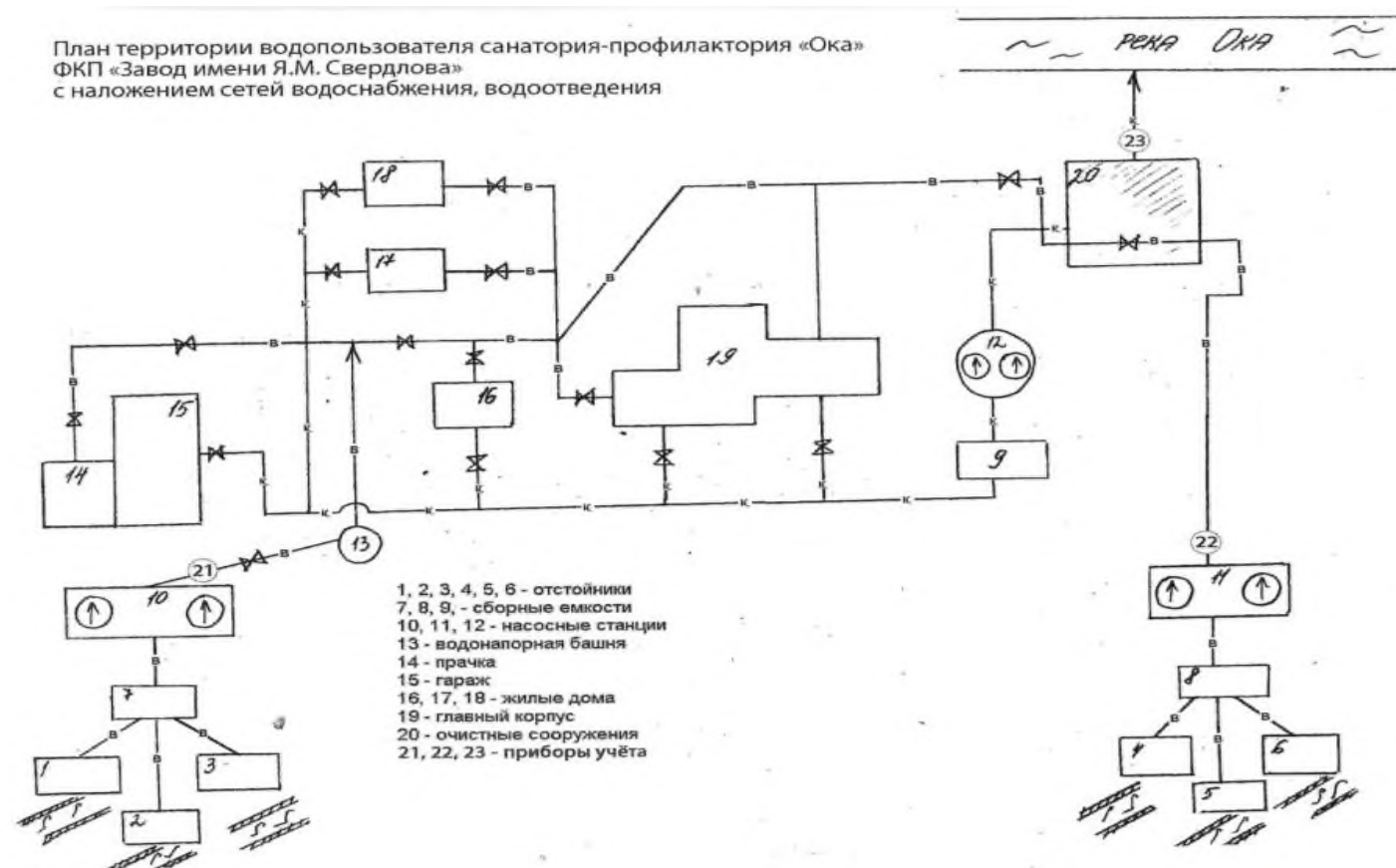
Схема 1 План территории водопользователя Санаторий-профилакторий «Ока» ФКП «Завод имени Я.М.Свердлова». Сети водоснабжения и водоотведения.
